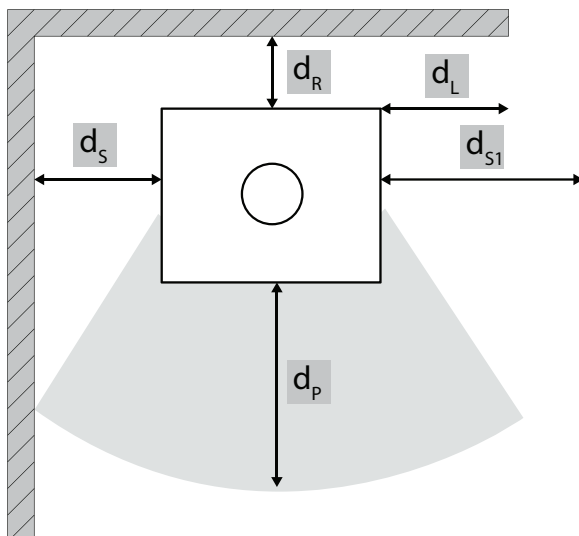
ODYN, ODYN L - ABSTÄNDE ZU BRENNBAREN STOFFEN; Positionsplan 1
